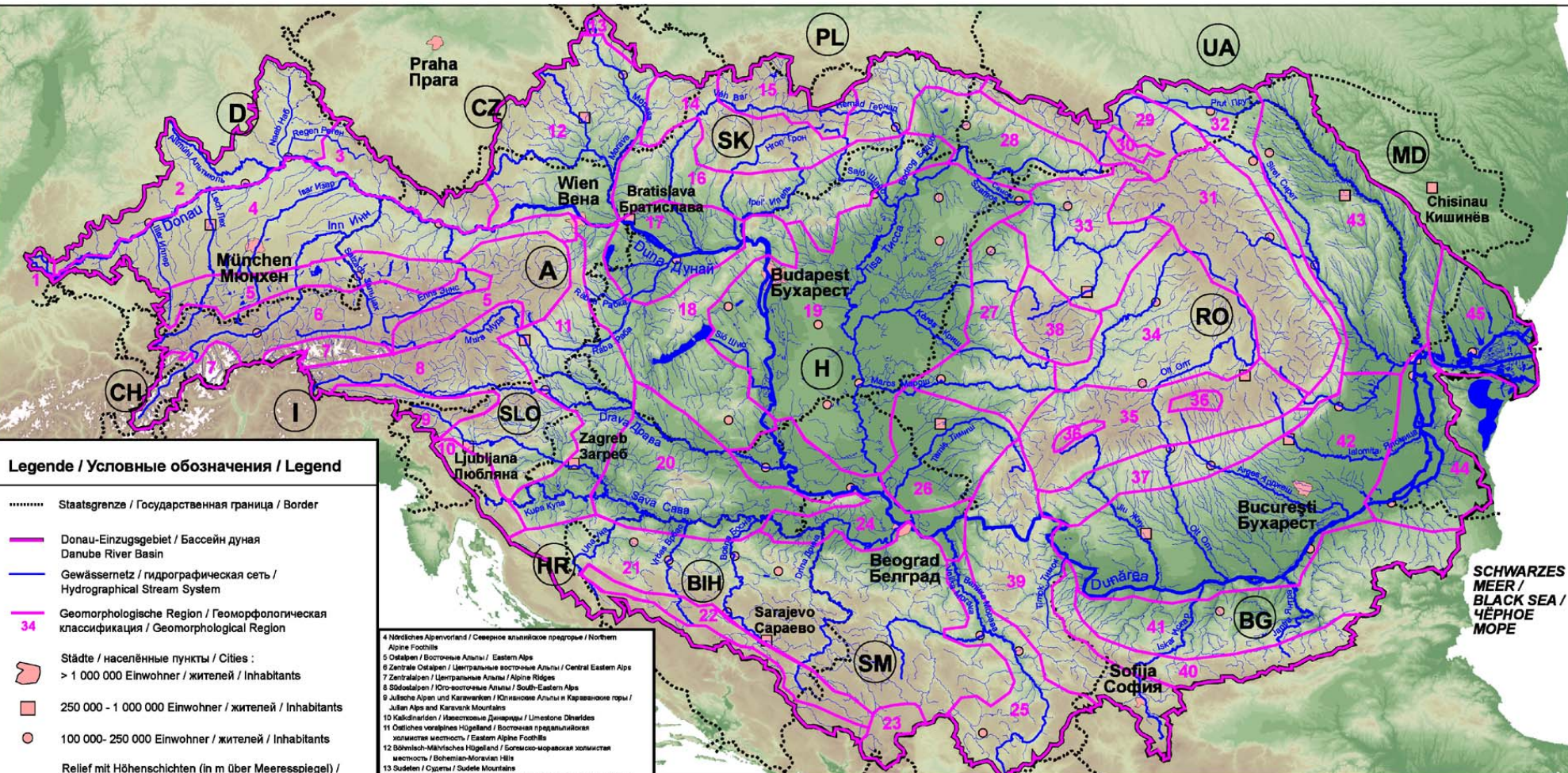
Karte 4: Donau-Einzugsgebiet - Geomorphologische Regionen und Gewässernetz / Карта 4: Бассейн Дуная - Геоморфологическая классификация и гидрографическая сеть / Map 4: Danube River Basin - Geomorphological Regions and Hydrographical Stream System
